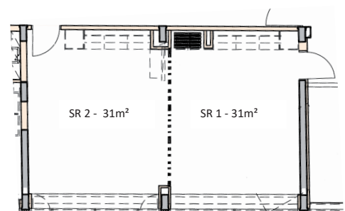
Skizze Raum ohne Trennwand (62m 2 )
